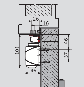
Угловая монтажная пластина для скользящего канала для установки на дверную раму с глубоким добором двери со стороны, противоположной петлям
