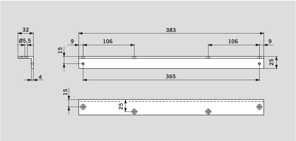
Угловая монтажная пластина для скользящего канала для установки на дверную раму с глубоким добором двери со стороны, противоположной петлям
